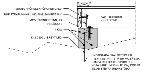
UPPBYGGING SÖKKLA UNDIR GÓLFGRIND HÚSS mkv. 1:10
