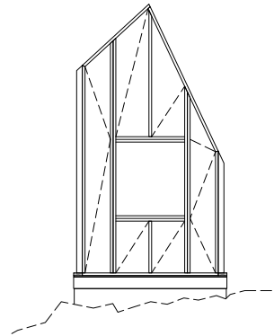
VEGGJAGRIND NORDVESTUR mkv. 1:50
