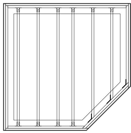
GRUNNMYND GÓLFGRINDAR mkv. 1:20
