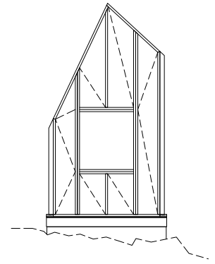
VEGGJAGRIND NORDAUSTUR mkv. 1:50
